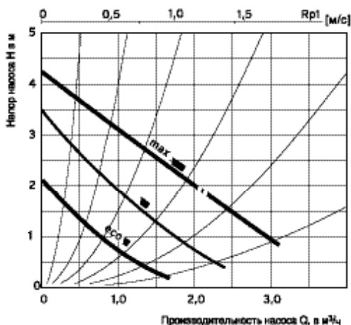
Рис. 14 Циркуляционный насос трёхступенчатый
