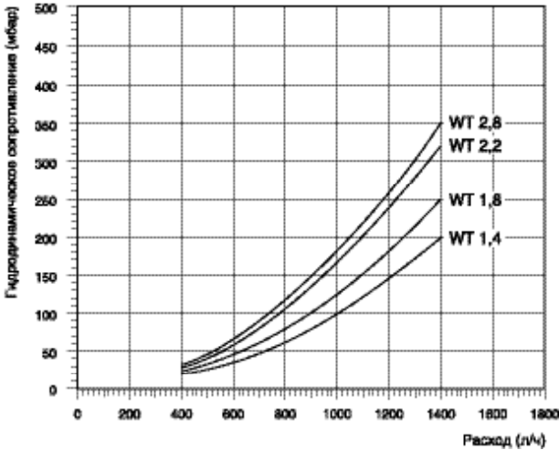
Потеря давления солнечного теплообменника VIN U 500
