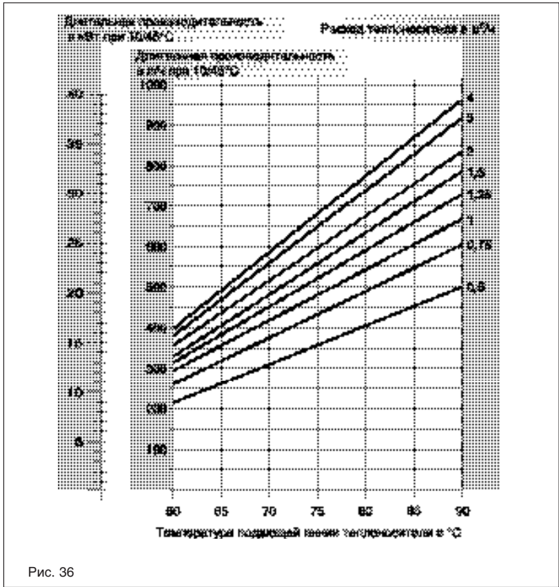
Длительная производительность VIN H 150
