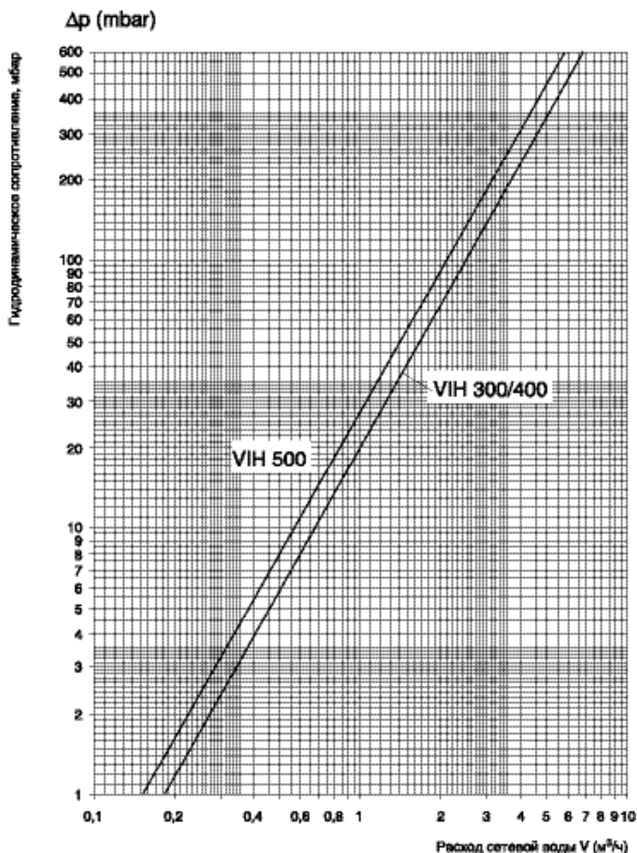
Рис. 52 Гидродинамическое сопротивление VIH 300–500
