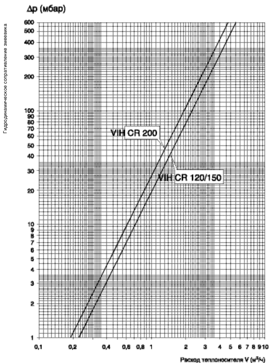
Рис. 47 Гидродинамическое сопротивление в змеевике VIH CR 120–200
