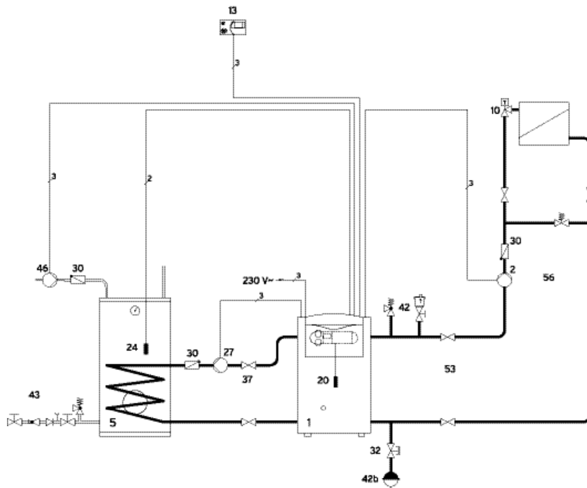
Рис. 16 Гидравлическая схема – Пример 1
