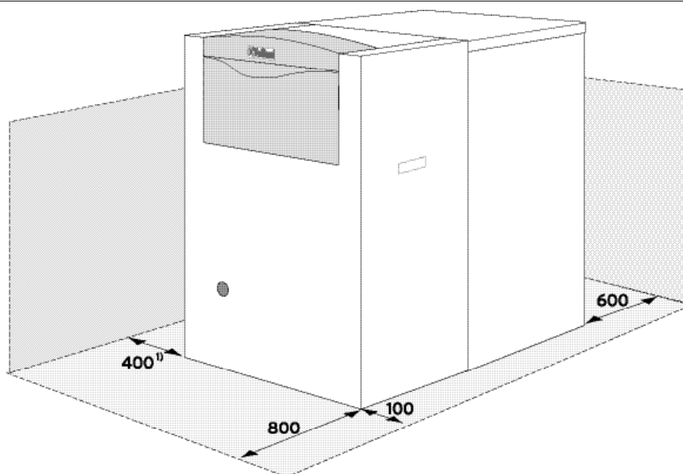
Рис. 11 Рекомендуемое минимальное расстояние между стенами для iroVIT VKO/VKO unit во время монтажных работ и работ по техническому обслуживанию Размеры в мм
