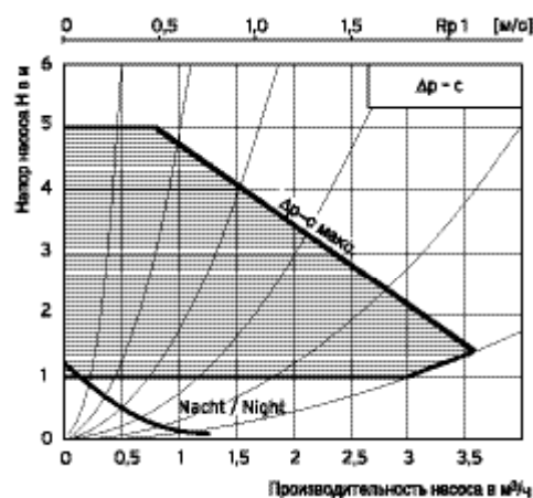
Рис. 12 Циркуляционный насос с электрическим регулированием, характеристика: Δp-постоянная
