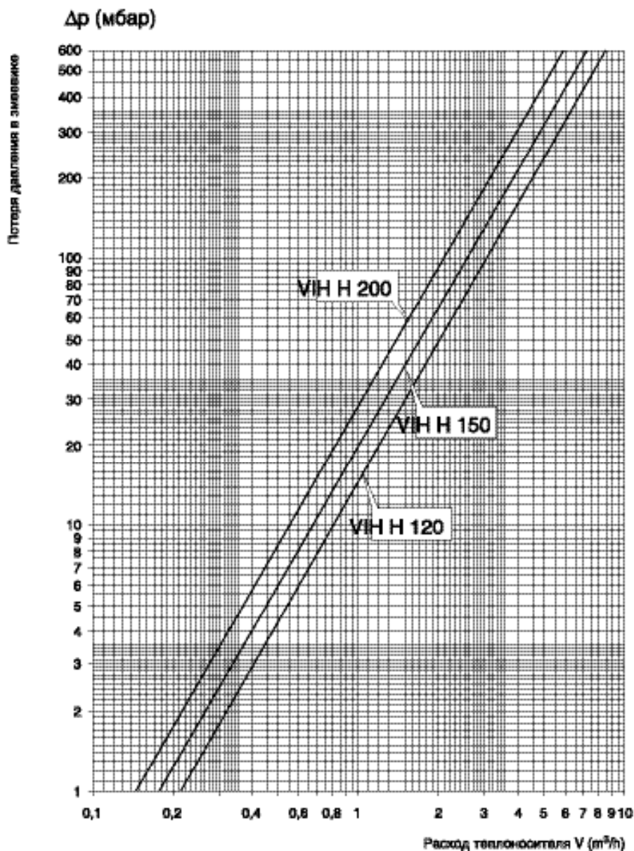
Рис. 40 Гидродинамическое сопротивление VIH H 120–200
