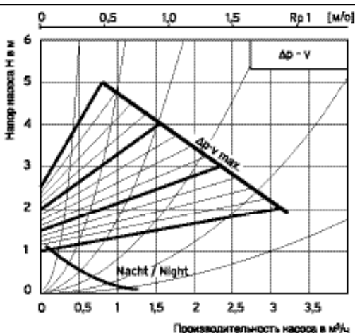
Рис. 13 Циркуляционный насос с электрическим регулированием, характеристика: Δp-переменная
