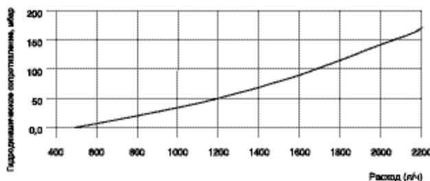
Потеря давления солнечного теплообменника VIH S 300/400
